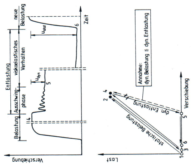
Abb. 3.9: Qualitatives Verschiebungs- (Extensometer/Fundamente) und Steifigkeitsverhalten (Untergrund)
