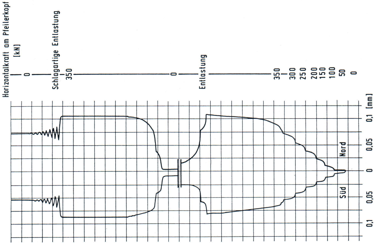
Abb. 2.8: Beispiele für Meßschriebe der Extensometerbewegungen
