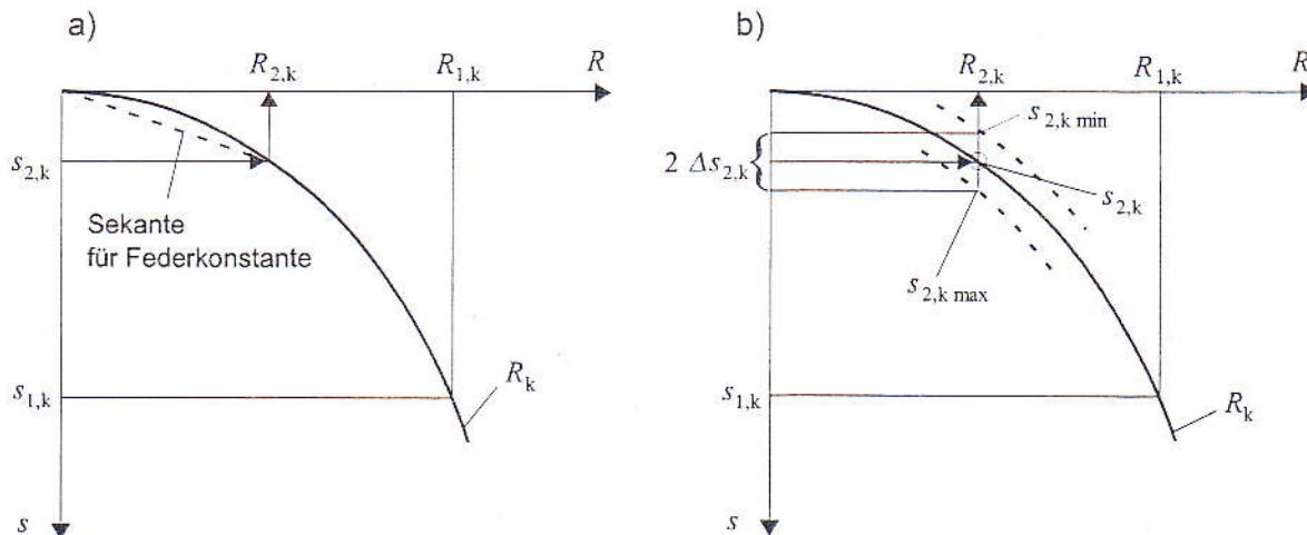
Bild 2: Ableitung der Pfahlwiderstände R_2 abhängig davon, ob geringe oder erhebliche Setzungsdifferenzen zu erwarten sind nach DIN 1054: 2003-01: a) bei zu erwartenden geringen Setzungsdifferenzen zwischen den Pfählen oder Pfahlgruppen, b) bei zu erwartenden erheblichen Setzungsdifferenzen zwischen den Pfählen oder Pfahlgruppen
