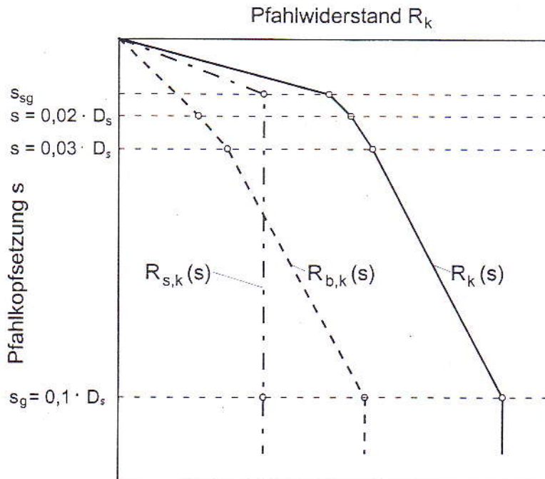
Bild 1: Elemente der charakteristischen Widerstands-Setzungslinie für Bohrpfähle, aus DIN 1054: 2003-01; für Pfähle mit Fußverbreiterung wird D s zu D b
