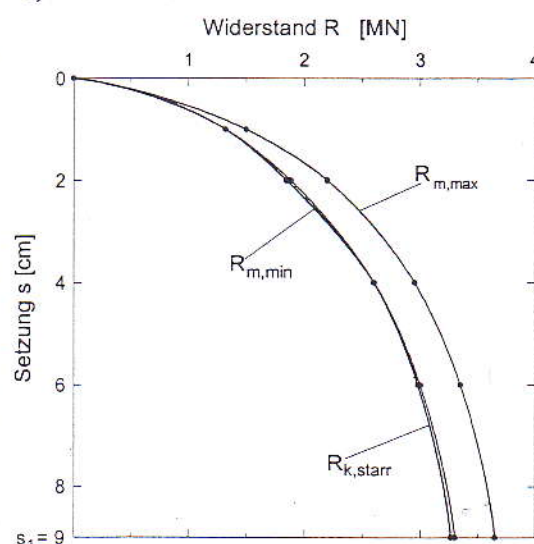
Bild 3: Beispiel zur Ableitung der charakteristischen WSL aus Pfahlprobelastungen a) System und Beanspruchung b) Ableitung nach DIN 1054: 2003-01 ohne Lastverteilung (weiches System) c) Ableitung nach DIN 1054: 2003-01 mit Lastverteilung (starres System)
