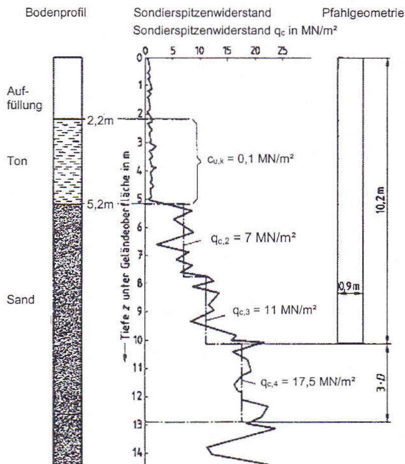
Bild 5: Bodenprofil, Sondierdiagramm und Maße für ein Anwendungsbeispiel zur Ermittlung der Widerstandssetzungslinie
