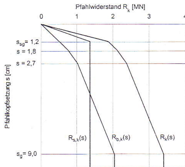
Bild 6: Widerstands-Setzungslinie
