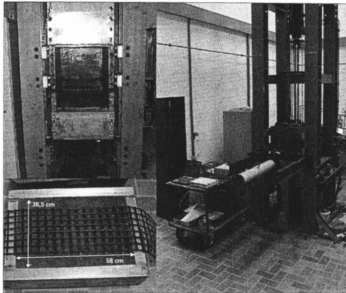
Bild 6: Großrahmenscherversuchsstand – Konfiguration für die Herauszieh- und Überlappungsversuche
