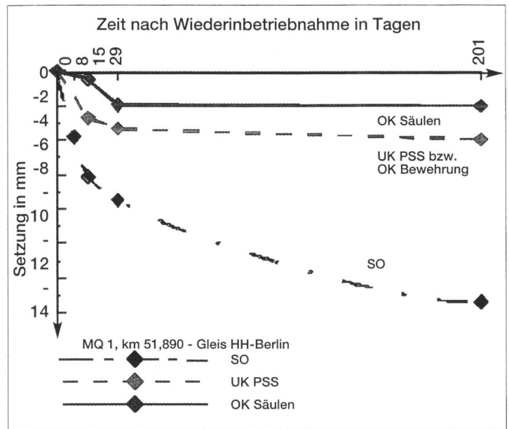
Bild 12: Setzungsverlauf im MQ1 in unterschiedlichen Höhen, Gleis Hamburg-Berlin
