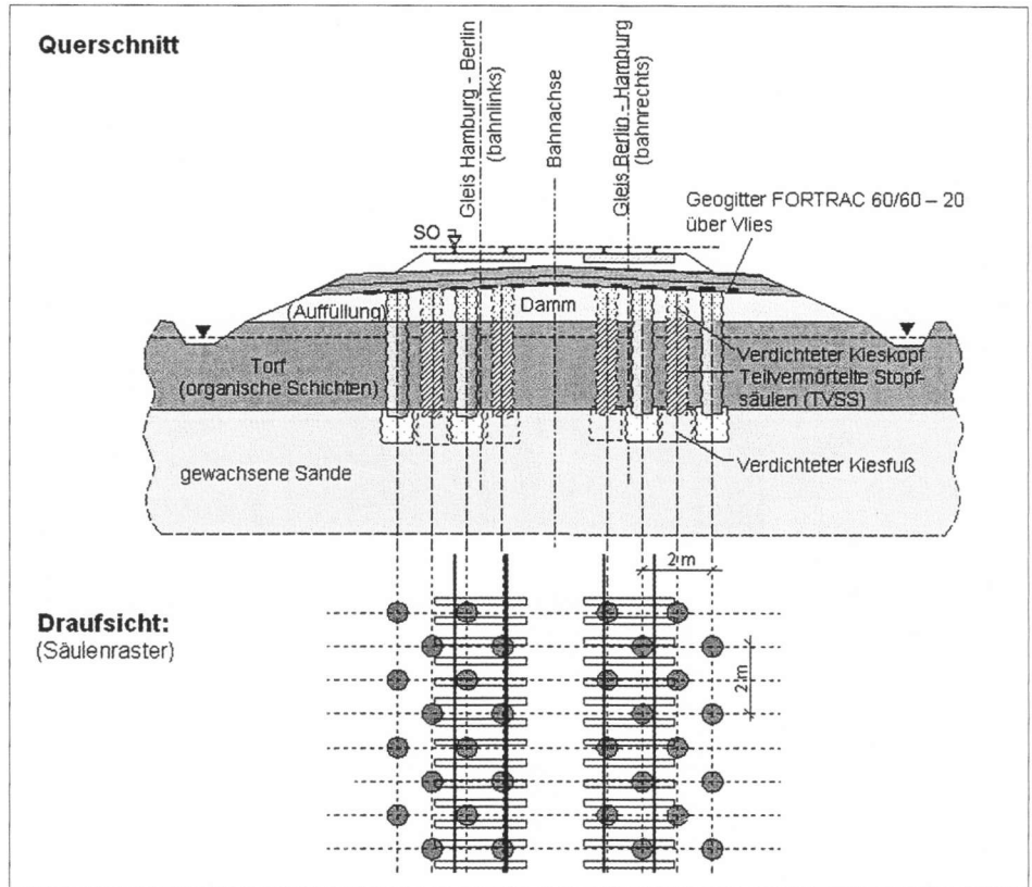
Bild 2: Querschnitt und Draufsicht nach der 1. Ausbaustufe
