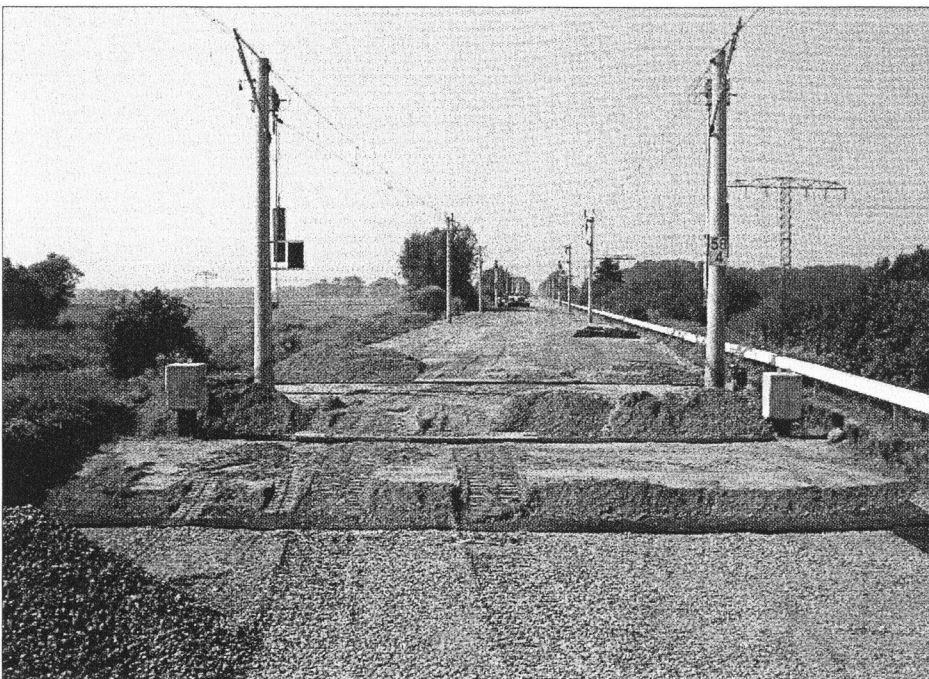
Bild 10: Einbau von Geogittern zwischen Paulineau und Friesack (Quelle: Tost, Arge PRA 1)
