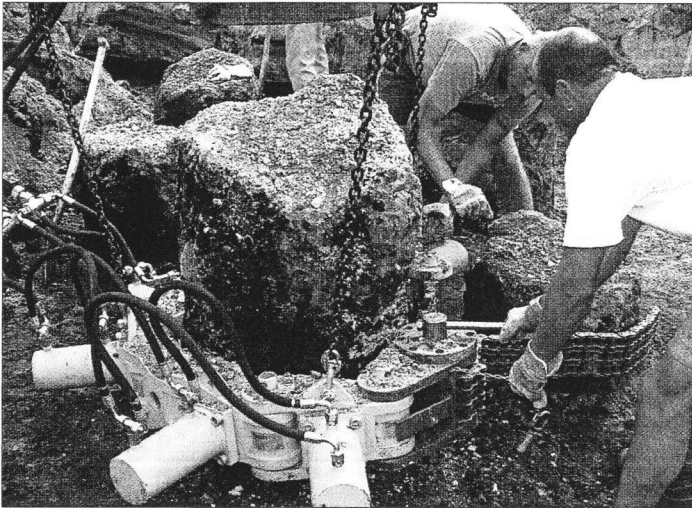
Bild 8: Schonendes Kürzen der TVSS
