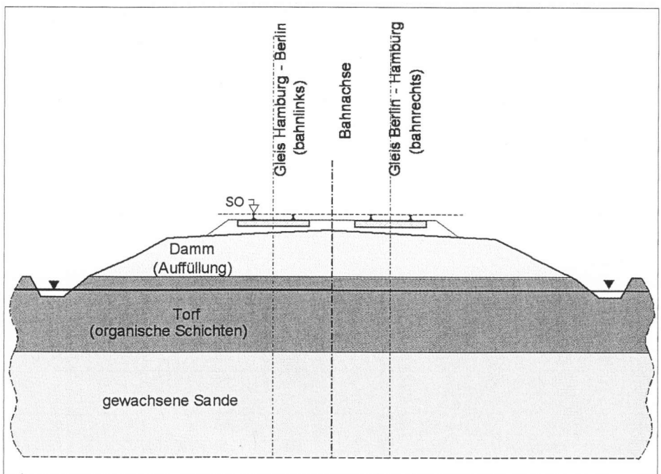
Bild 1: Typische Baugrundsituation vor der 1. Ausbaustufe
