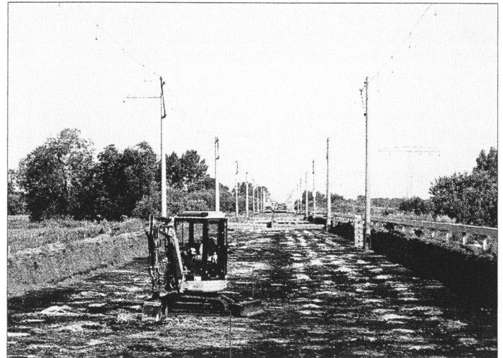
Bild 9: Abtragsniveau bei -2,7 m unter SO
