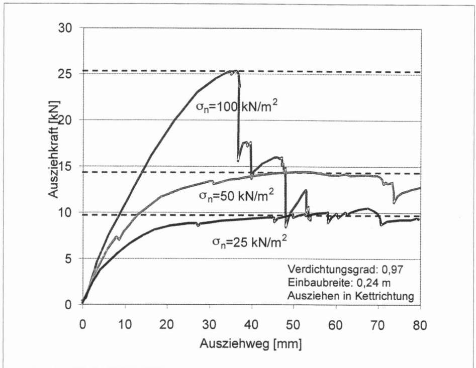
Bild 7: Exemplarisches Versuchsergebnis: Herausziehversuch für D_{Pr} = 0,97
