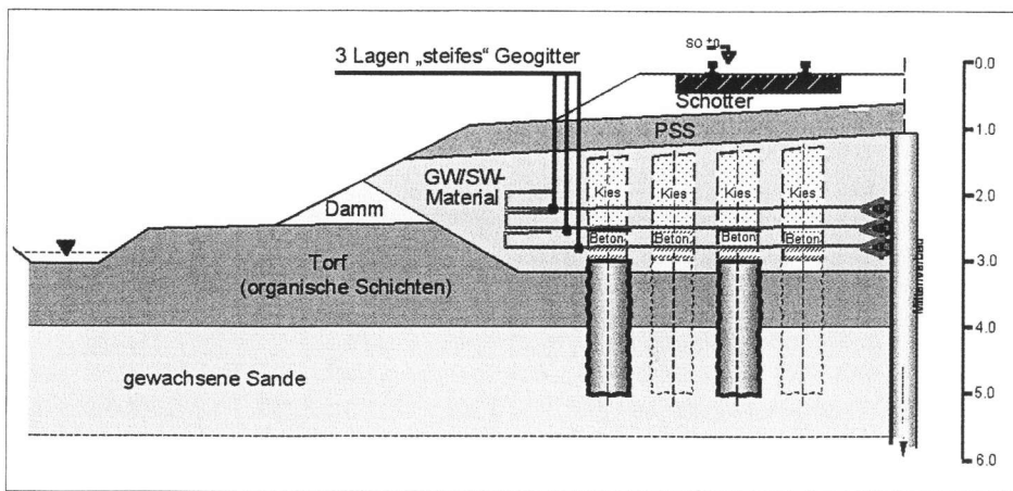
Bild 4: Regelquerschnitt der Ausschreibung zur Tragsystemertüchtigung
