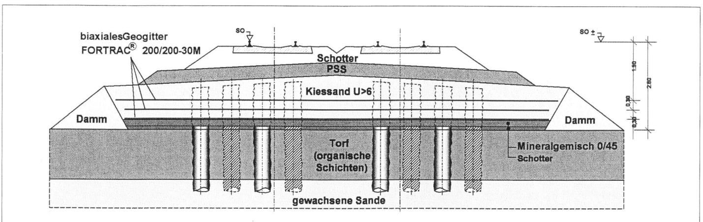
Bild 5: Querschnitt des ausgeführten Tragsystems
